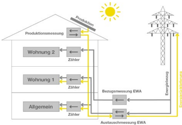
Abbildung 2: Messgeräteanordnung 2
