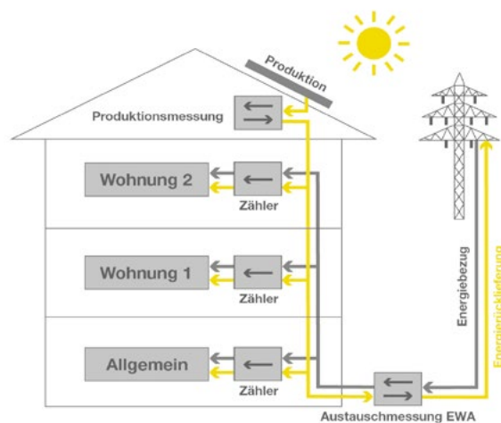
Abbildung 1: Messgeräteanordnung 1
